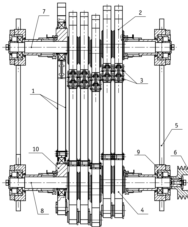
Рис. 8. Главный узел станка (динамически сбалансированный пильный блок): 1 – пильные полотна (общее количество – 6, 12, 18 шт.), 2 – верхний шарнирный узел с элементами подвижной фиксации пильного полотна и корректирующей массой, 3 – упругие элементы, 4 – нижний шарнирный узел с элементами крепления пильного полотна и корректирующей массой, 5 – боковая стойка, 6 – шкив нижнего вала пильного блока, 7 – верхний вал, 8 – нижний вал, 9 – подшипниковые опоры валов, 10 – эксцентрик
