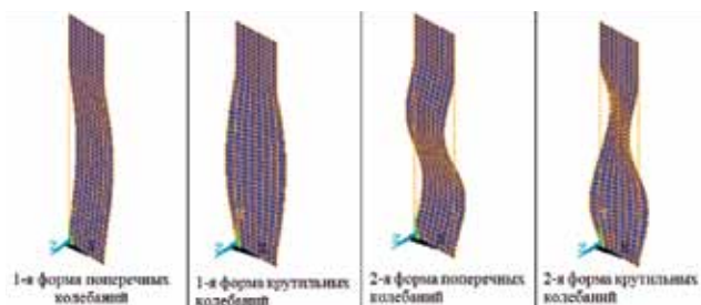
Рис. 4. Поведение пильных полотен: различные формы собственных колебаний пильных полотен шириной 80 мм, длиной 350 мм и толщиной 1,47 мм
