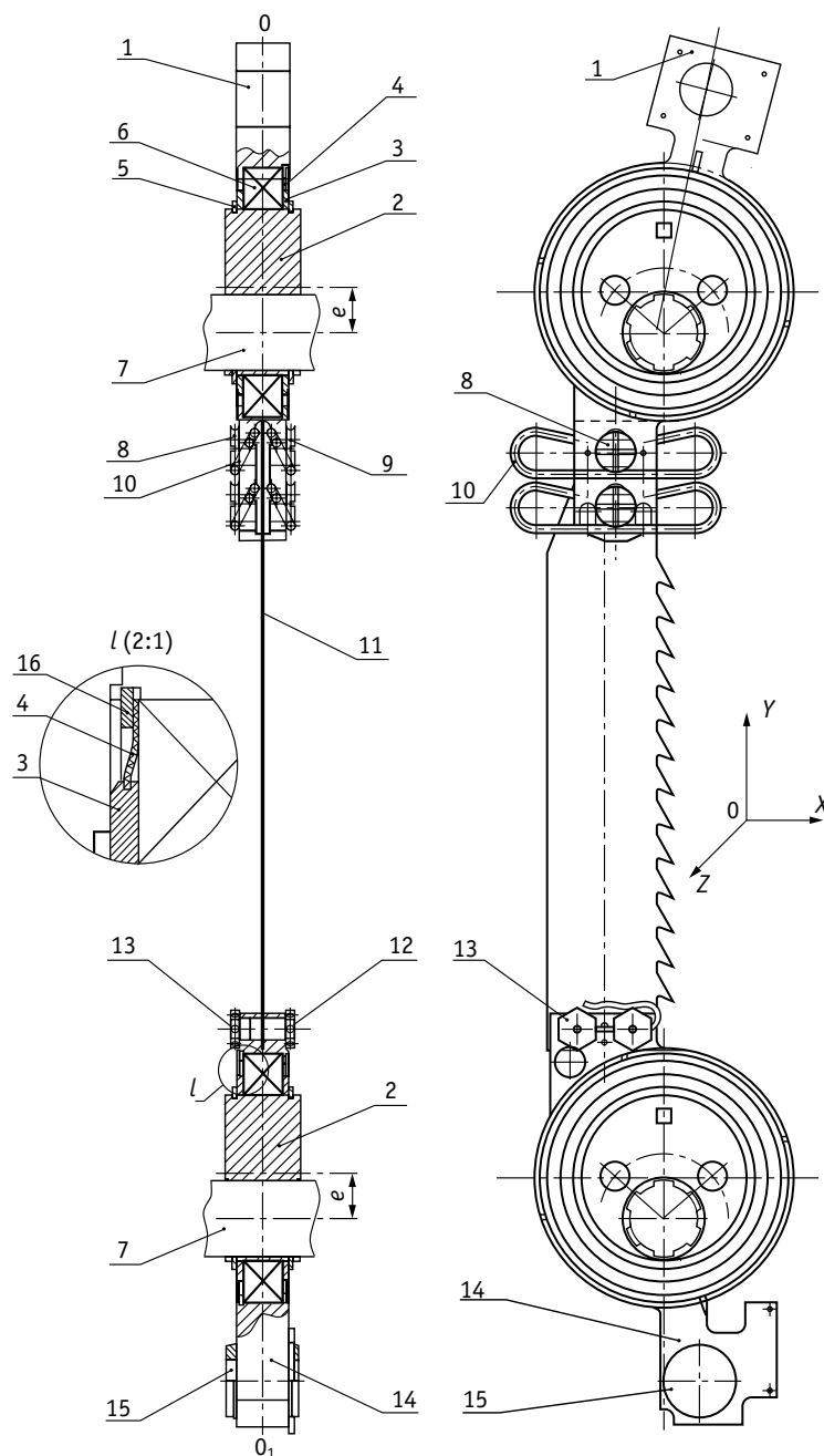
Рис. 6. Главный узел пильного блока: 1 – верхний шарнирный узел, 2 – эксцентрик, 3 – кольцо, 4 – кольцо пыльник, 5 – пружинное кольцо (запорное), 6 – радиально-упорный подшипник, 7 – вал шлицевой, 8, 9 – крепеж верхнего шарнирного узла, 10 – упругий элемент (скоба), 11 – пильное полотно, 12, 13 – крепеж нижнего шарнирного узла, 14 – нижний шарнирный узел, 15 – устройство баланса (корректирующая масса) со шпилькой, 16 – пружинное кольцо (запорное)
