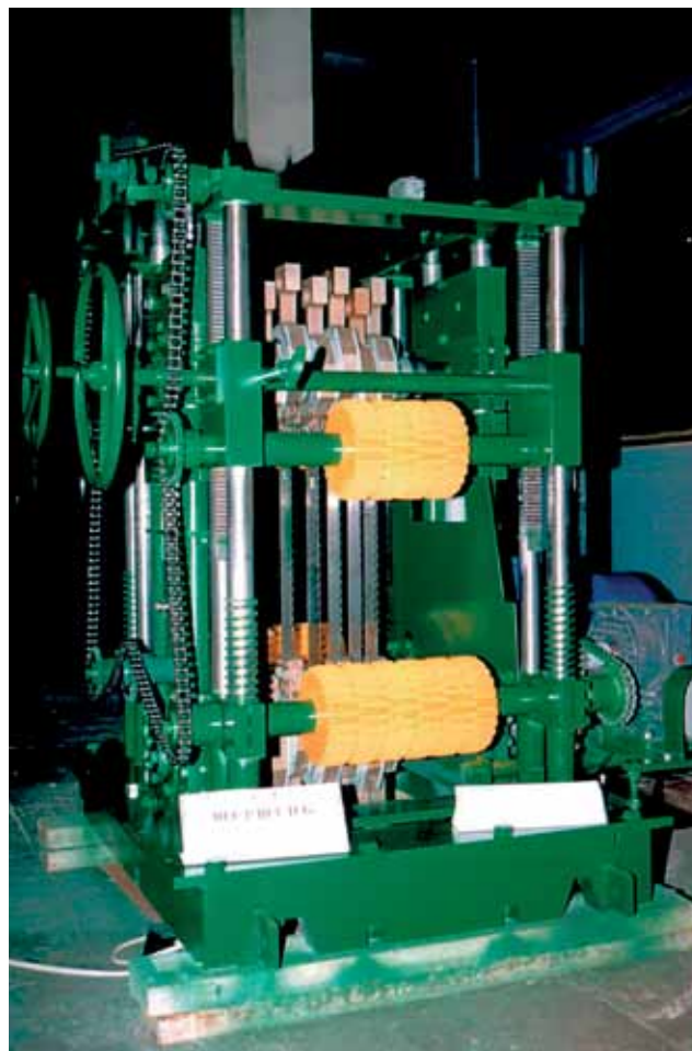
Рис. 2. Станок модели М2001 (без кожуха) для распиловки бревен
